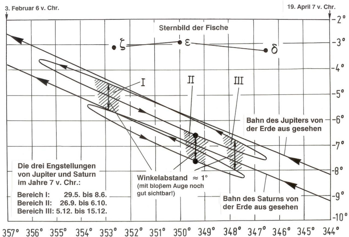
Bild 5: Von der Erde aus gesehen führen die Bahnen von Jupiter und Saturn Schleifenbewegungen aus. Bei der dreifachen Konjunktion von Jupiter und Saturn im Jahre 7 v. Chr. betrug selbst in den drei Zeiten der Annäherung (I, II und III) der Abstand ein Grad, und das sind zwei Vollmonddurchmesser.
